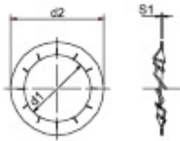
Forma J – Dentado Interno
