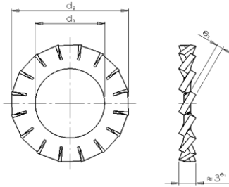
Forma A – Dentado Externo
